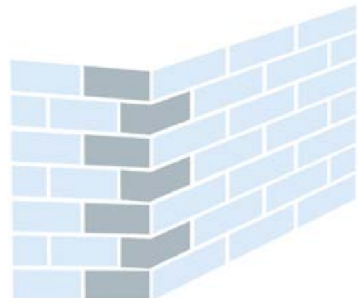
SCHNITT GERADE an Ecke
