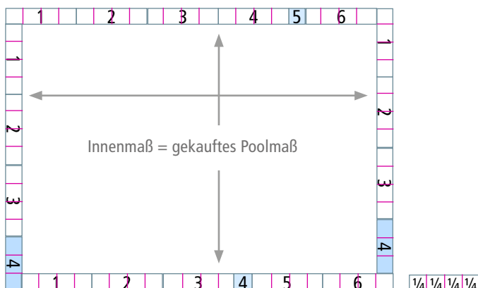
DRAUFSICHT Beispiel: Styroporpool 500 x 350 cm
